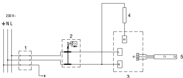
SI. 5: Električna spojna shema
