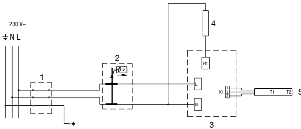
Bild 5: Elektroschaltbild
