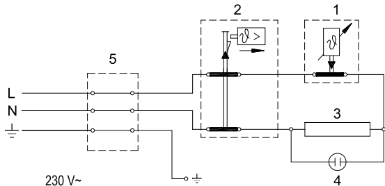
Elektroschaltbild
