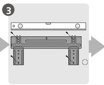
Pričvrstite ploču za montažu
