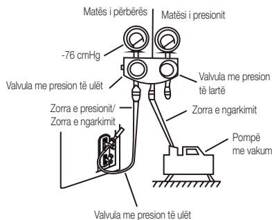
Manometër (matës i shumëfishtë)
